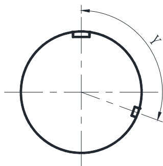
插座（从正面看）
